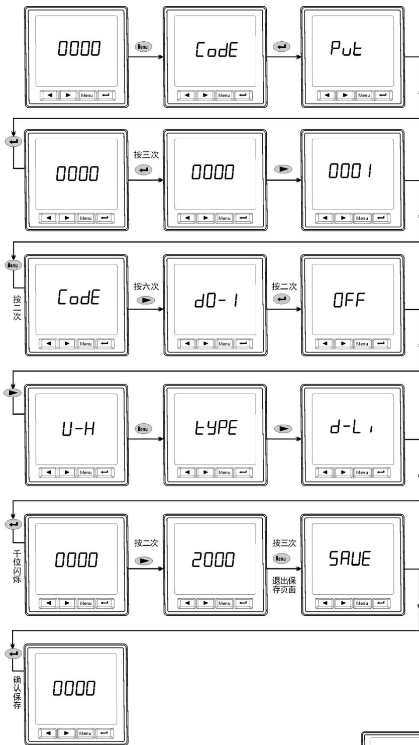
例 4：报警输出设置（例：设定 D01，电压高于 200V 报警）
